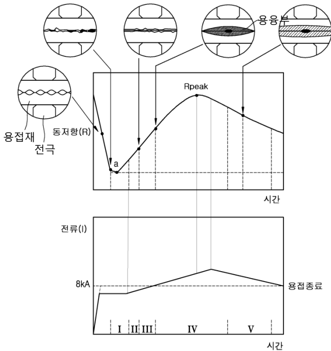
[본 기술에 따른 시간별 전류량공급과 용접형태를 도시한 그림]
