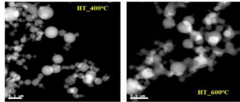
[본 기술에 따른 Ni-W 나노 입자의 STEM-EDS 성분 분석 결과]
