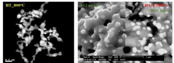
[본 기술에 따른 Ni-W 나노 입자를 열처리하였을 때 형상 변화]
