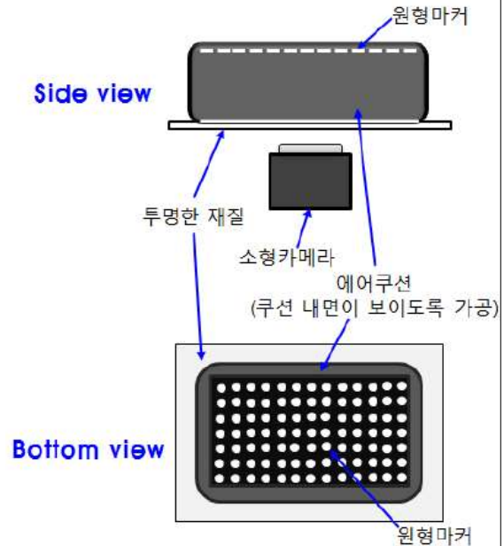
[하드웨어 구성도]
